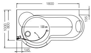
TWINLINE 1 Badewanne 180
