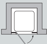
Tür in Nische mit 2 Fixteilen
